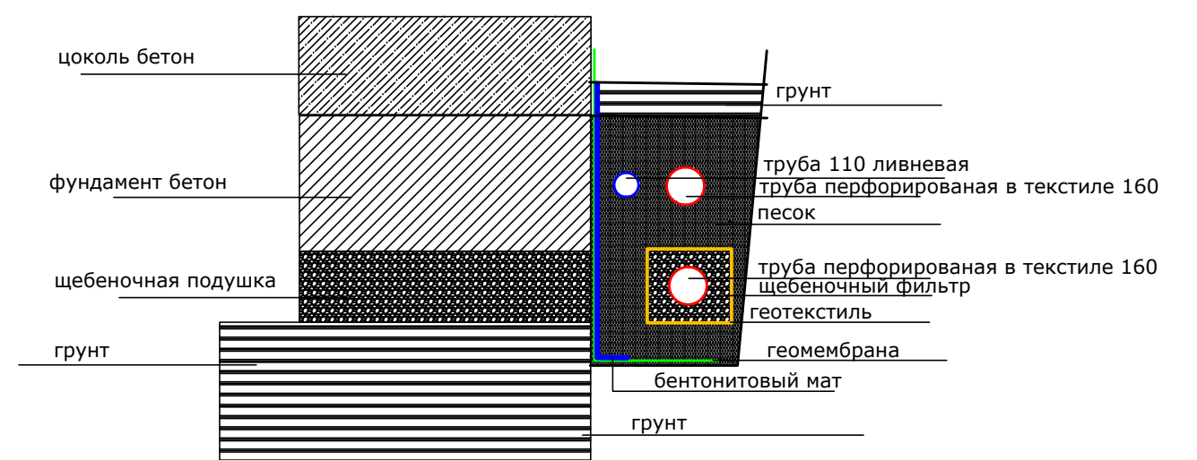
Разрез прифундаментной траншеи
